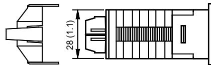
Vue de derrière avec le cadre de fixation
