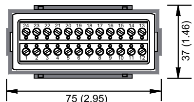
Vue de derrière avec le cadre de fixation
