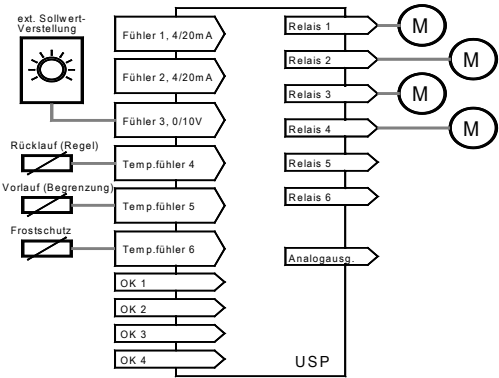
Kaltwasserregler mit 4 Einzelmaschinen, externe Sollwertverstellung über Normsignal oder Potentiometer.
